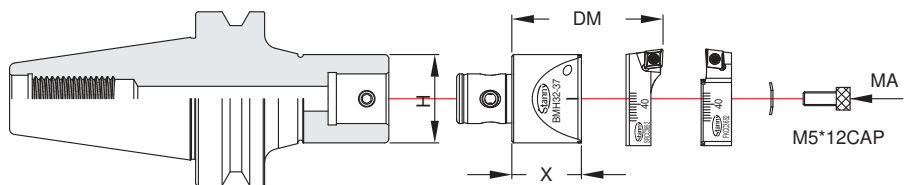
接桿 Shank
