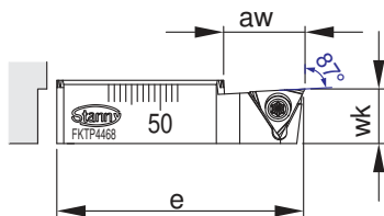
精搪孔反搪刀座 Reverse Cutting Insert Holder
