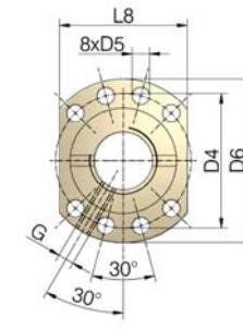
Hole pattern 2 to DIN 69051
