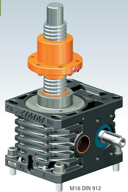
M16 DIN 912
