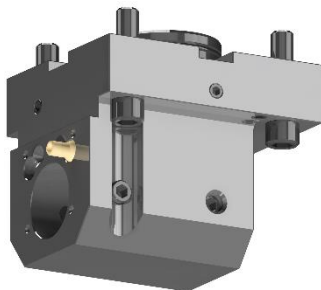
NGT ID-60x40x80(MS)
